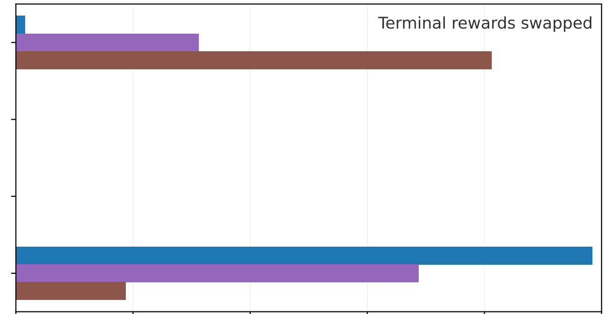
V2_Navigate
