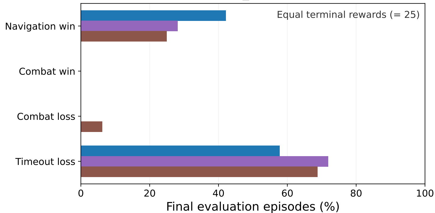
V1_Base
